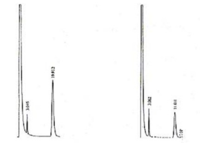
图A 标准品气相色谱图 图B 片剂试样气相色谱图 图中 t_r=0.588 溶剂， 图中 t_r=0.6 溶剂， t_r=3.045 大蒜辣素 t_r=3.062 大蒜辣素 t_r=11.011 大蒜素 t_r=10.912 大蒜素
